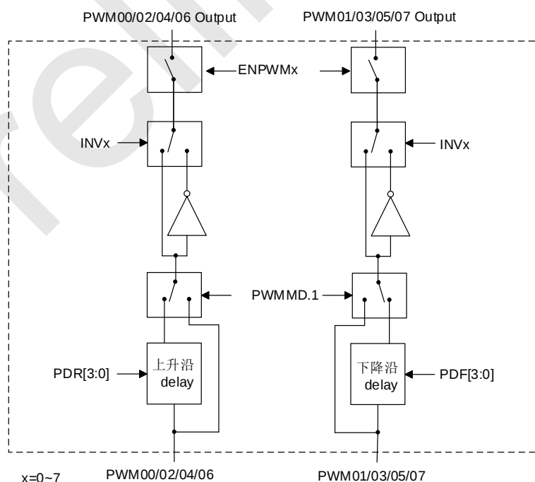
SC92F531X PWM 互补模式框图
